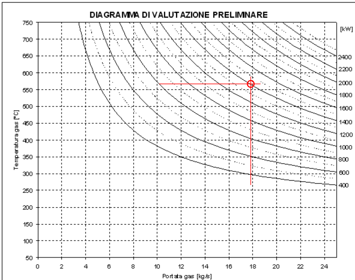
Diagramma di stima preliminare delle potenzialità di recupero con tecnologia ORC Turboden.
